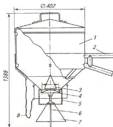
Рисунок 1. Кормушка клапанная
